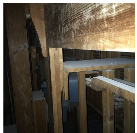
Orgelmotor sichtbar zwischen Balganlage und Orgelgehäuse
