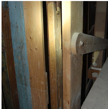
Detail der jetzigen Balganlage mit Spuren der alten Keilbalganlage links am Gehäuse Pfosten und hinten am Kanal
