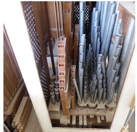
seitlicher Einblick in die Orgel: schwach sichtbar ichtbar die Aufdoppelung der Stöcke im Pedal links und im Manual rechts
